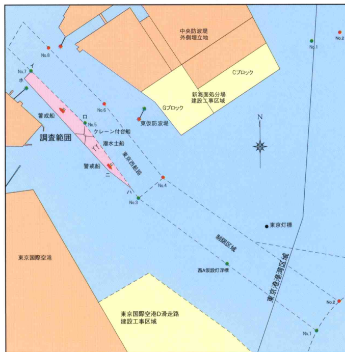
図-1 工事状況図
